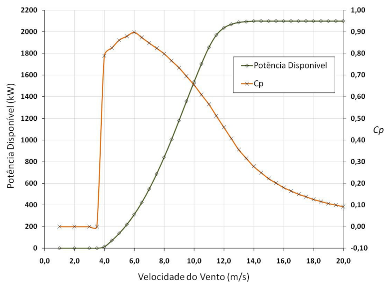
Figura 1. Curva de potência típica de uma aerogerador de 2,1 MW.
