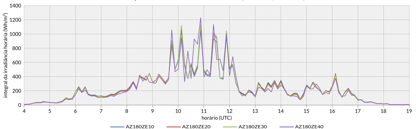
Espectrorradiômetro - dia 06/05/2017 (Hannover, Alemanha)
