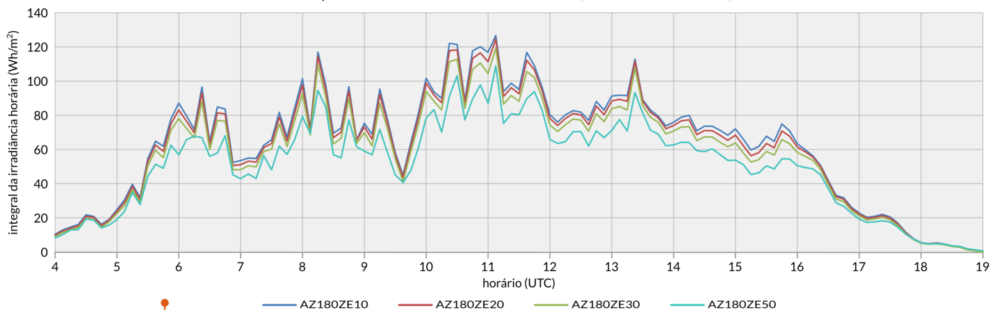
Espectrorradiômetro - dia 05/05/2017 (Hannover, Alemanha)
